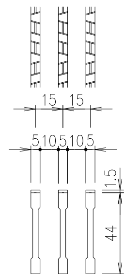
メインバー詳細図 S=1/2
