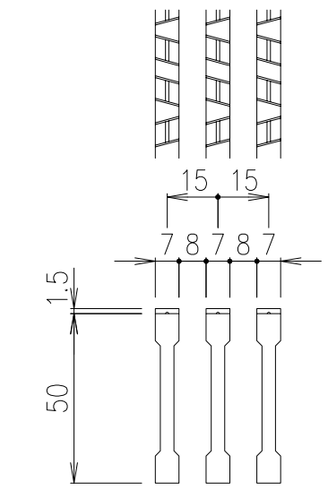
メインバー 詳細図 S=1/2
