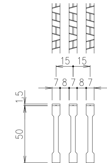
メインバー 詳細図 S=1/2
