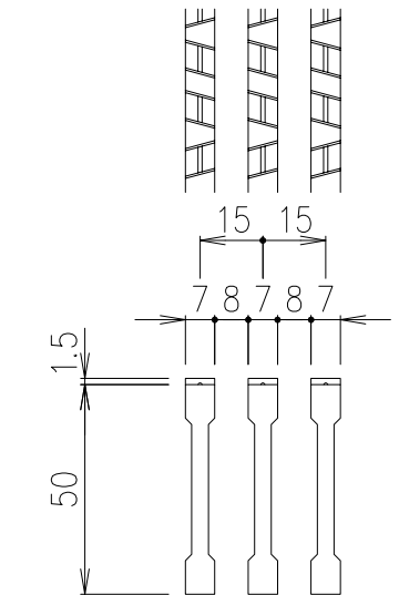
メンバー詳細図 S=1/2
