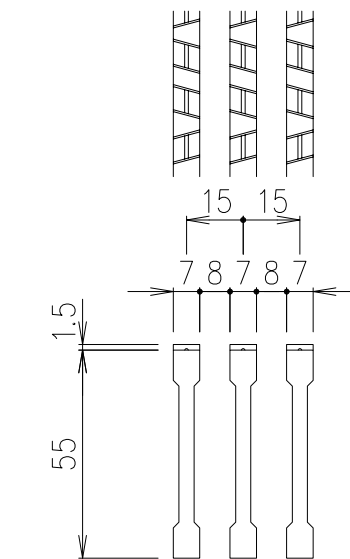
メインバー 詳細図 S=1/2
