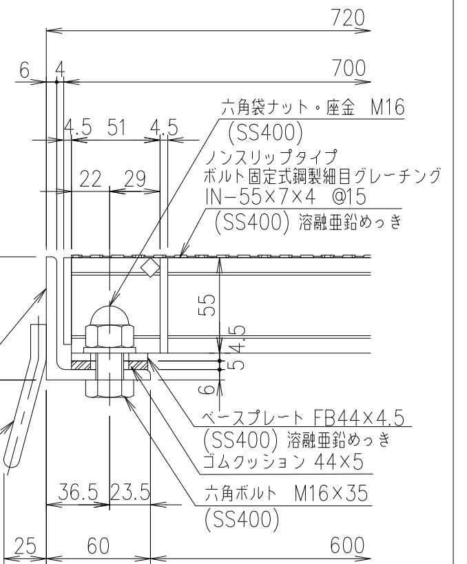
断面詳細図 S=1/3
