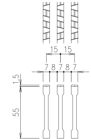
メンバー詳細図 S=1/2
