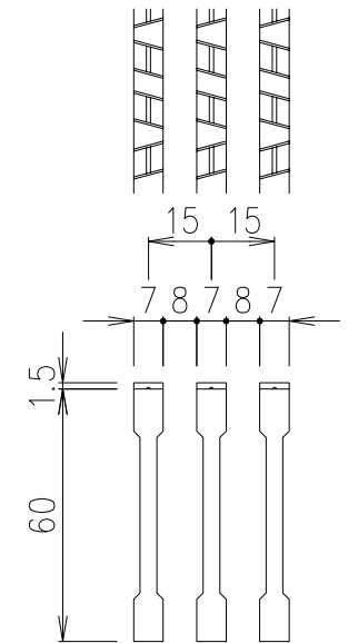
メンバー詳細図 S=1/2
