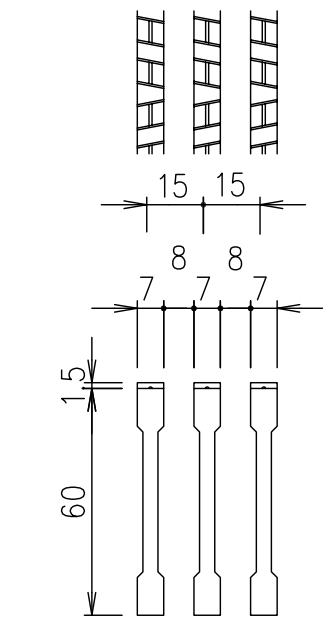
メインバー詳細図 S=1/2
