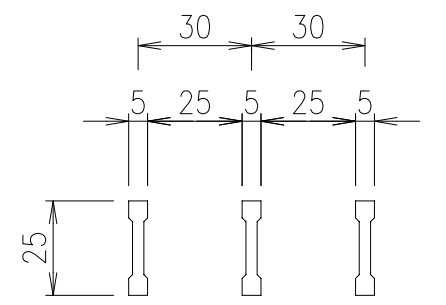
メインバー詳細図 S=1/2
