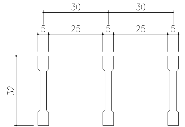
メインバーピッチ詳細図 S=1/1
