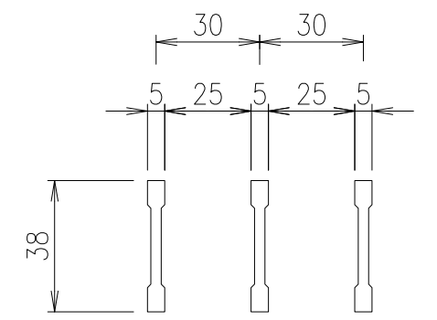
メインバー詳細図 S=1/2
