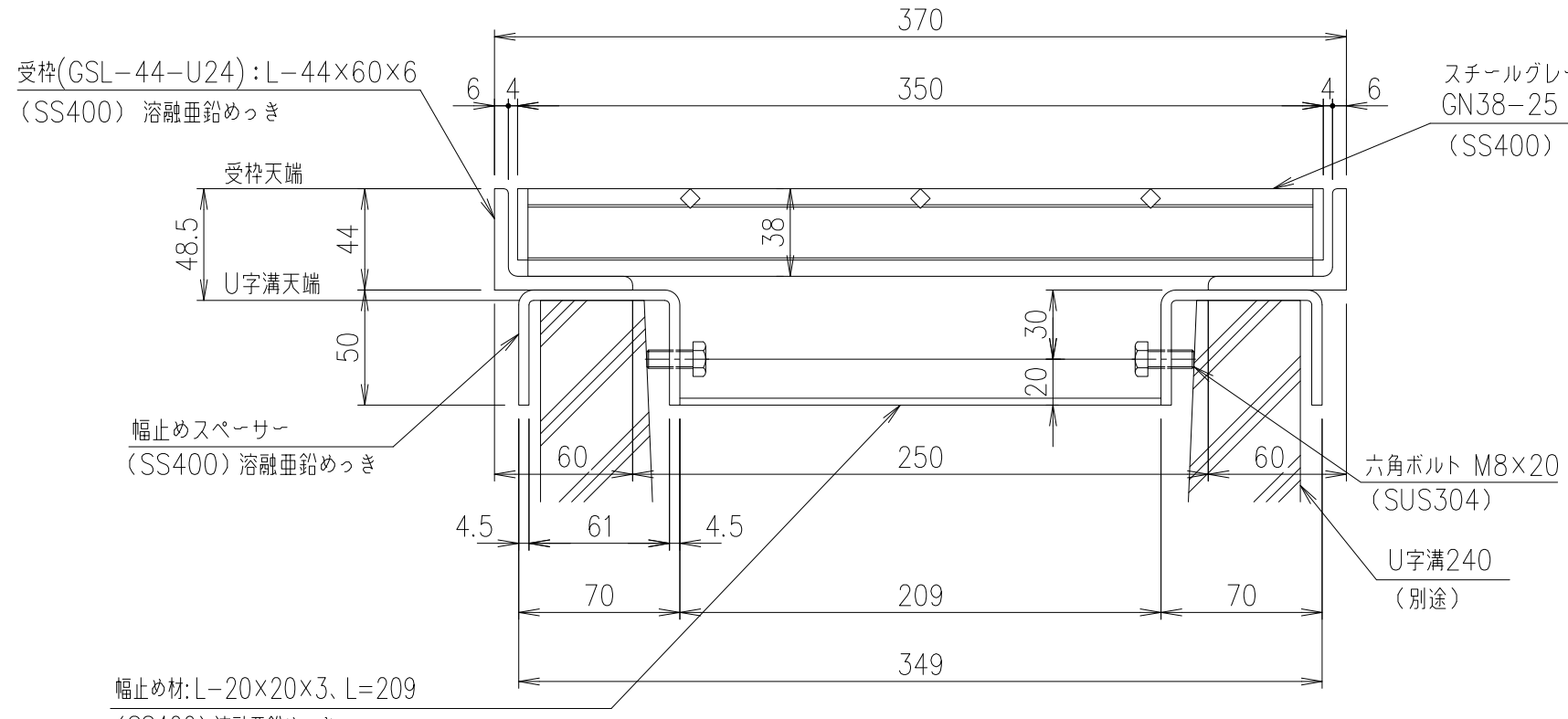
断面詳細図 S=1/3
