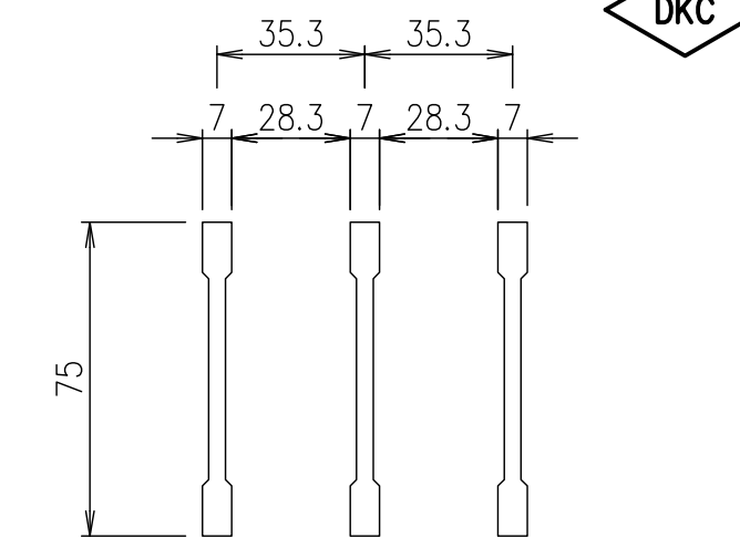
メインバー詳細図 S=1/2
