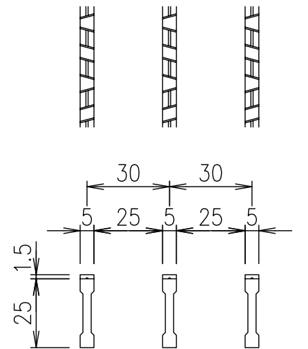
メインバー詳細図 S=1/2
