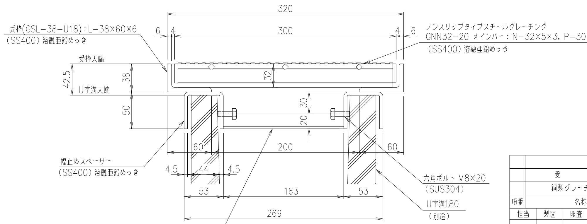
断面詳細図 S=1/3 幅止め材: L-20x20x3, L=163 (SS400) 溶融亜鉛めっき ※この幅止め材は、施工後も取り外さないでください。
