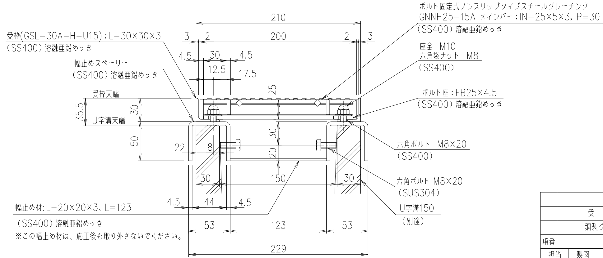
断面詳細図 S=1/3
