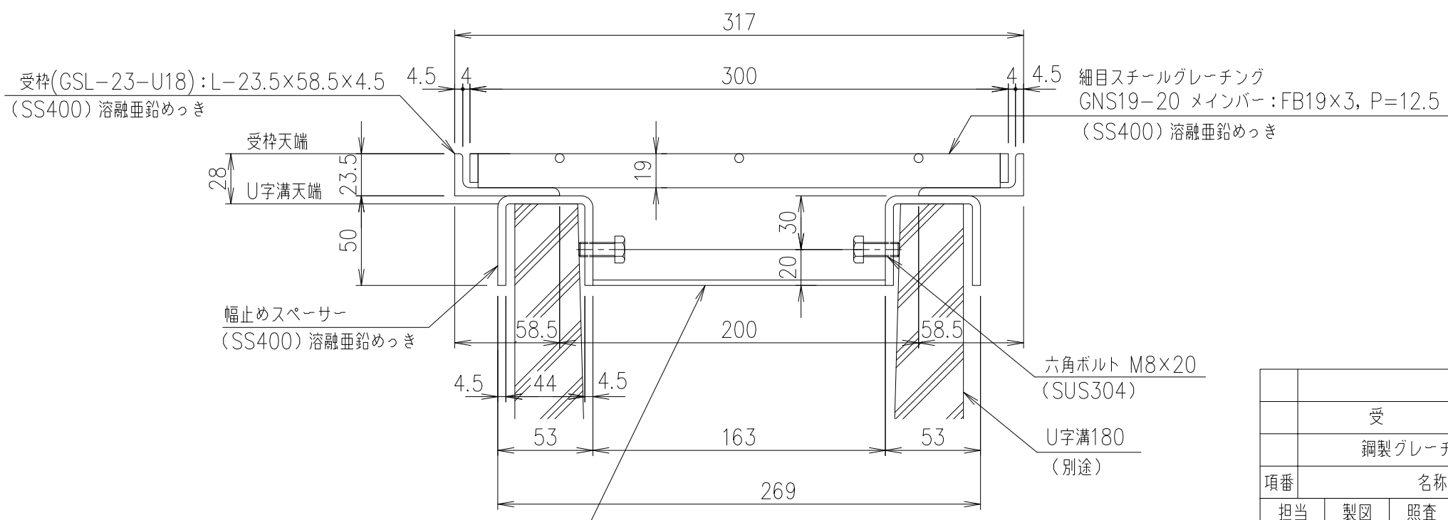
断面詳細図 S=1/3
