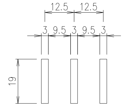
メインバー詳細図 S=1/1
