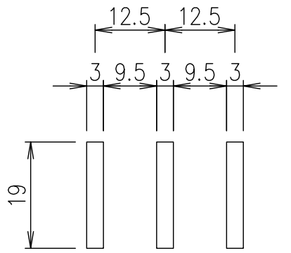
メインバー詳細図 S=1/1
