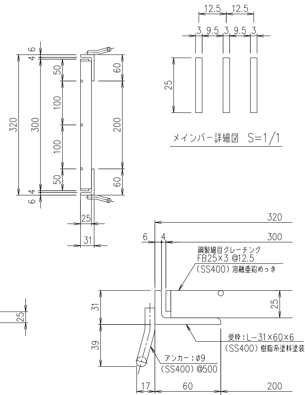
断面詳細図 S=1/2
