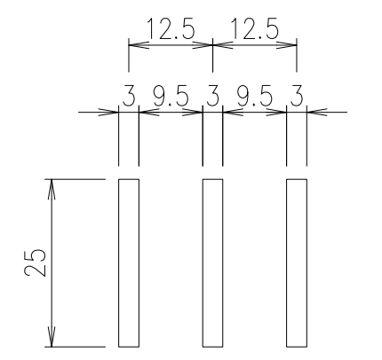
メインバー詳細図 S=1/1
