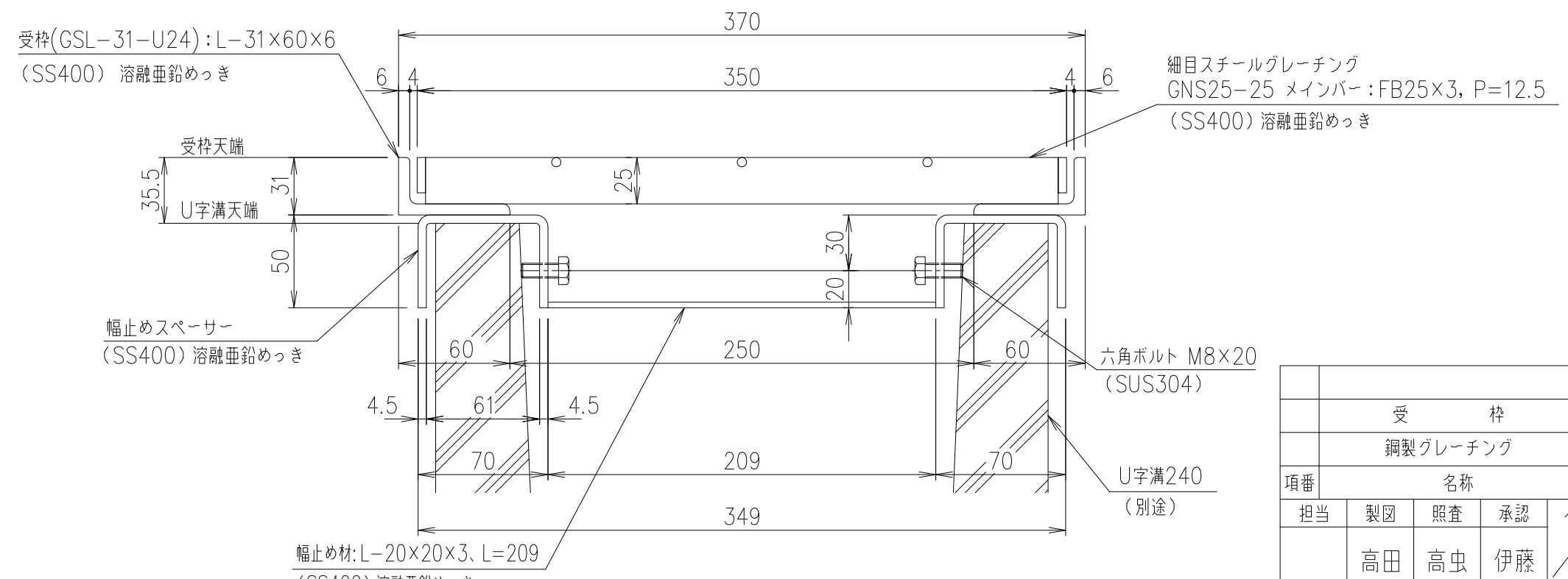
断面詳細図 S=1/3
