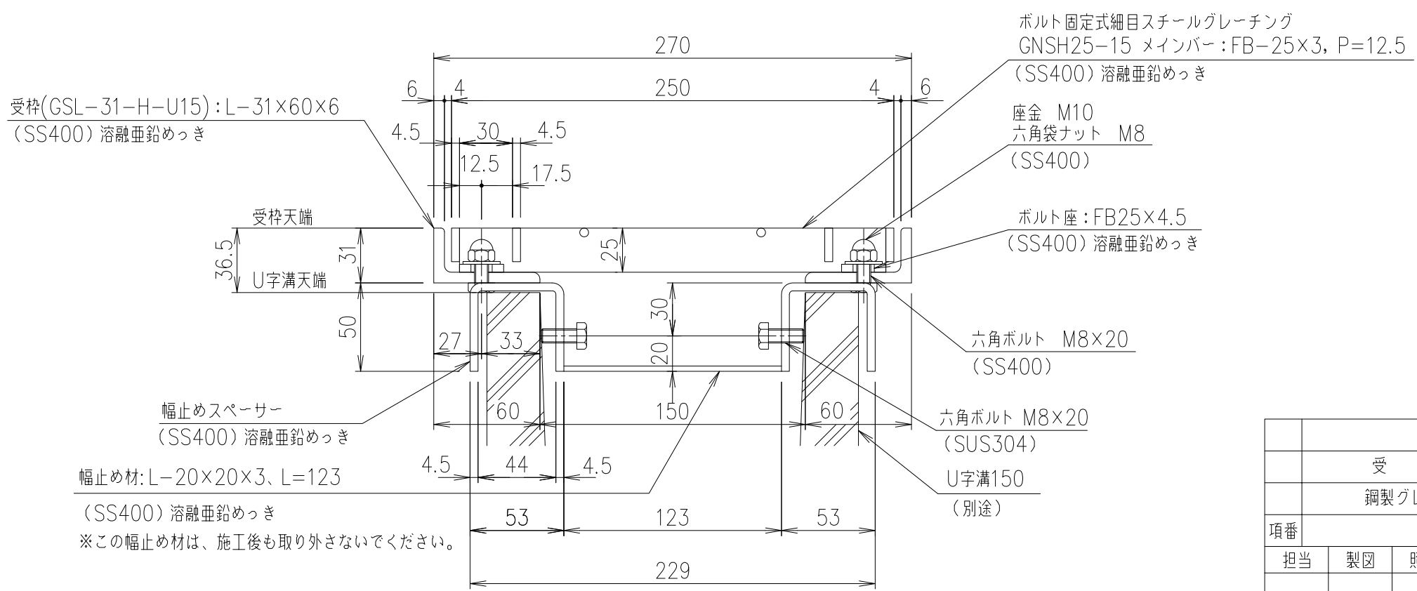
断面詳細図 S=1/3
