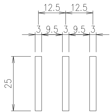
メインバー詳細図 S=1/1
