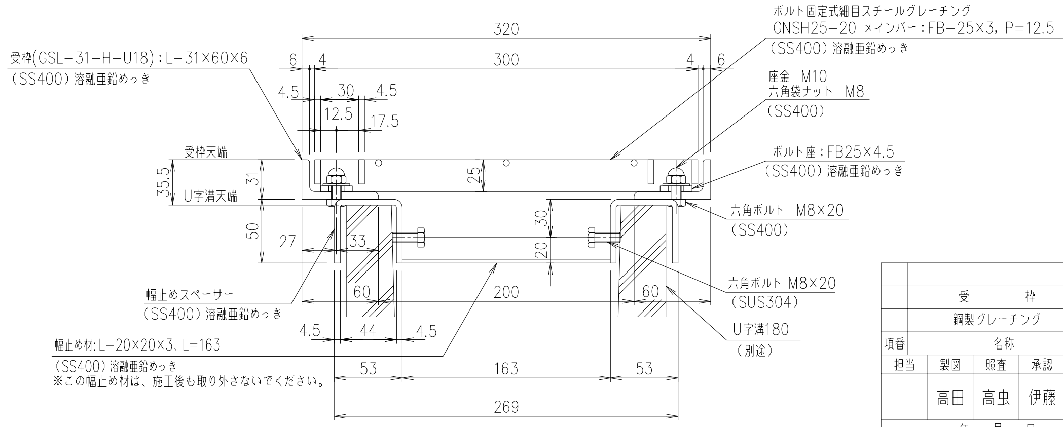
断面詳細図 S=1/3
