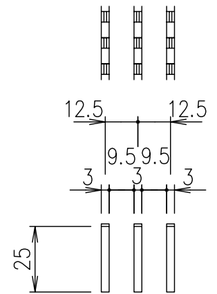
メンバー詳細図 S=1/2
