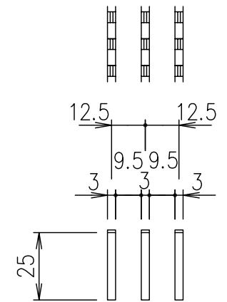
メンバー詳細図 S=1/2
