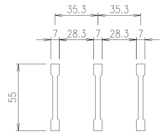
メンバー詳細図 S=1/2
