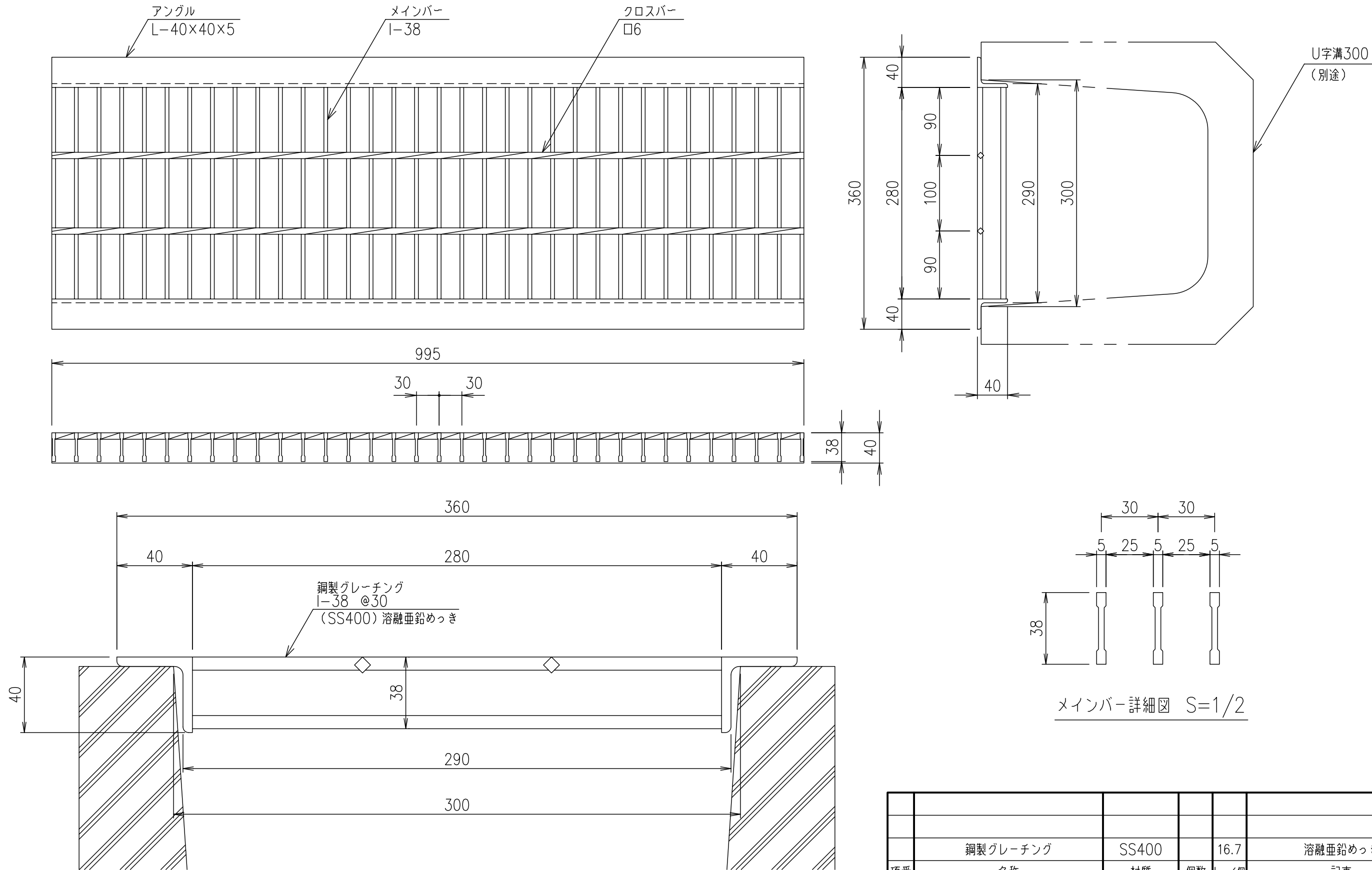
断面詳細図 S=1/2
