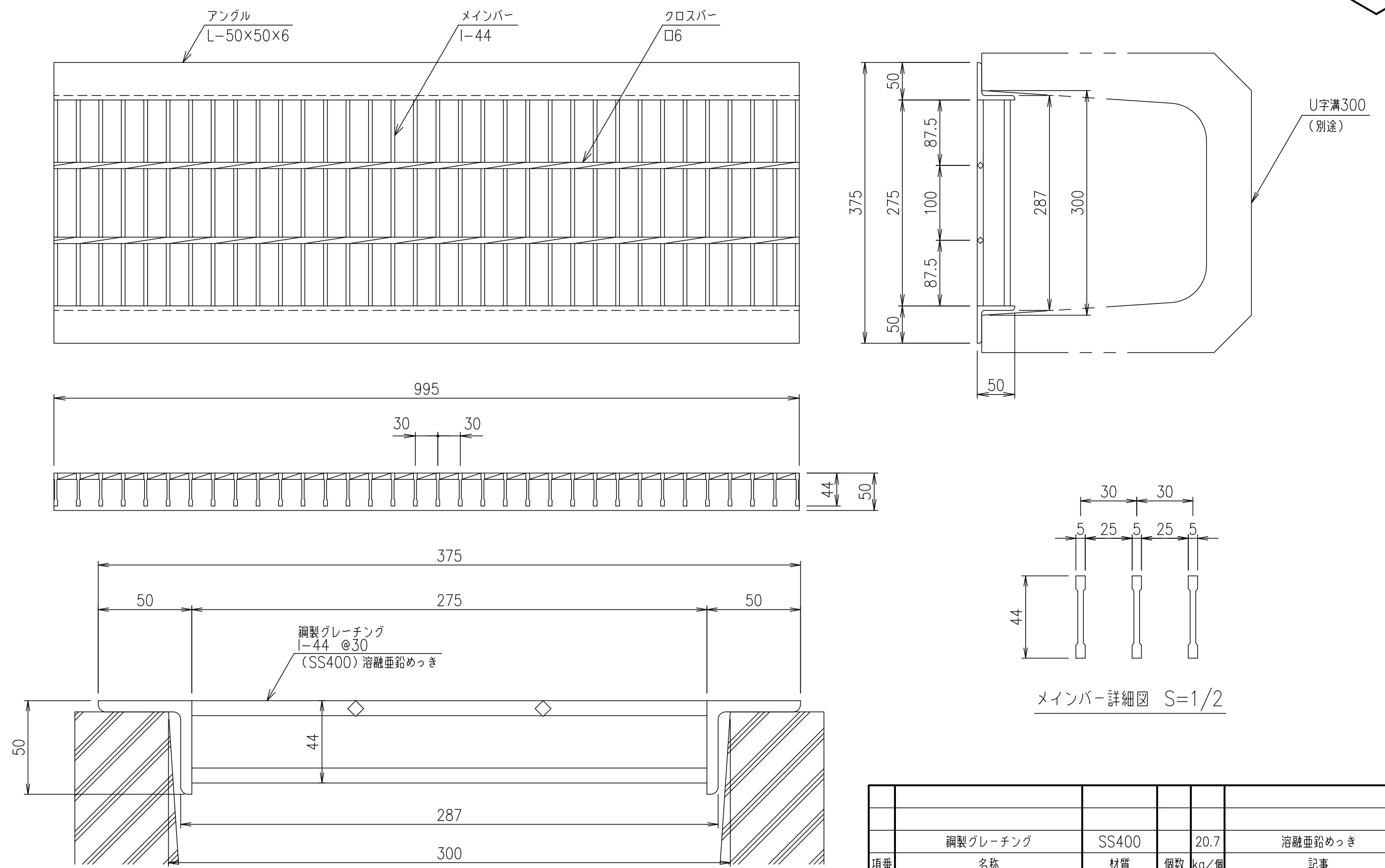
断面詳細図 S=1/2
