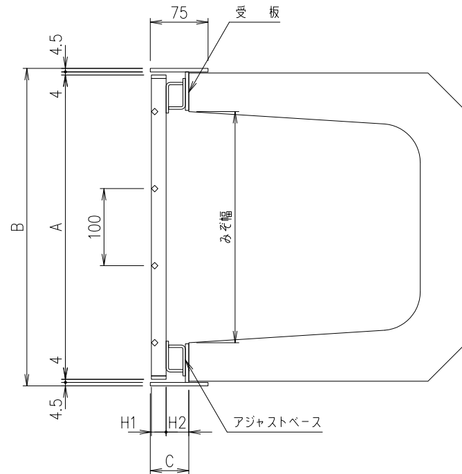
型式・寸法・材料表
