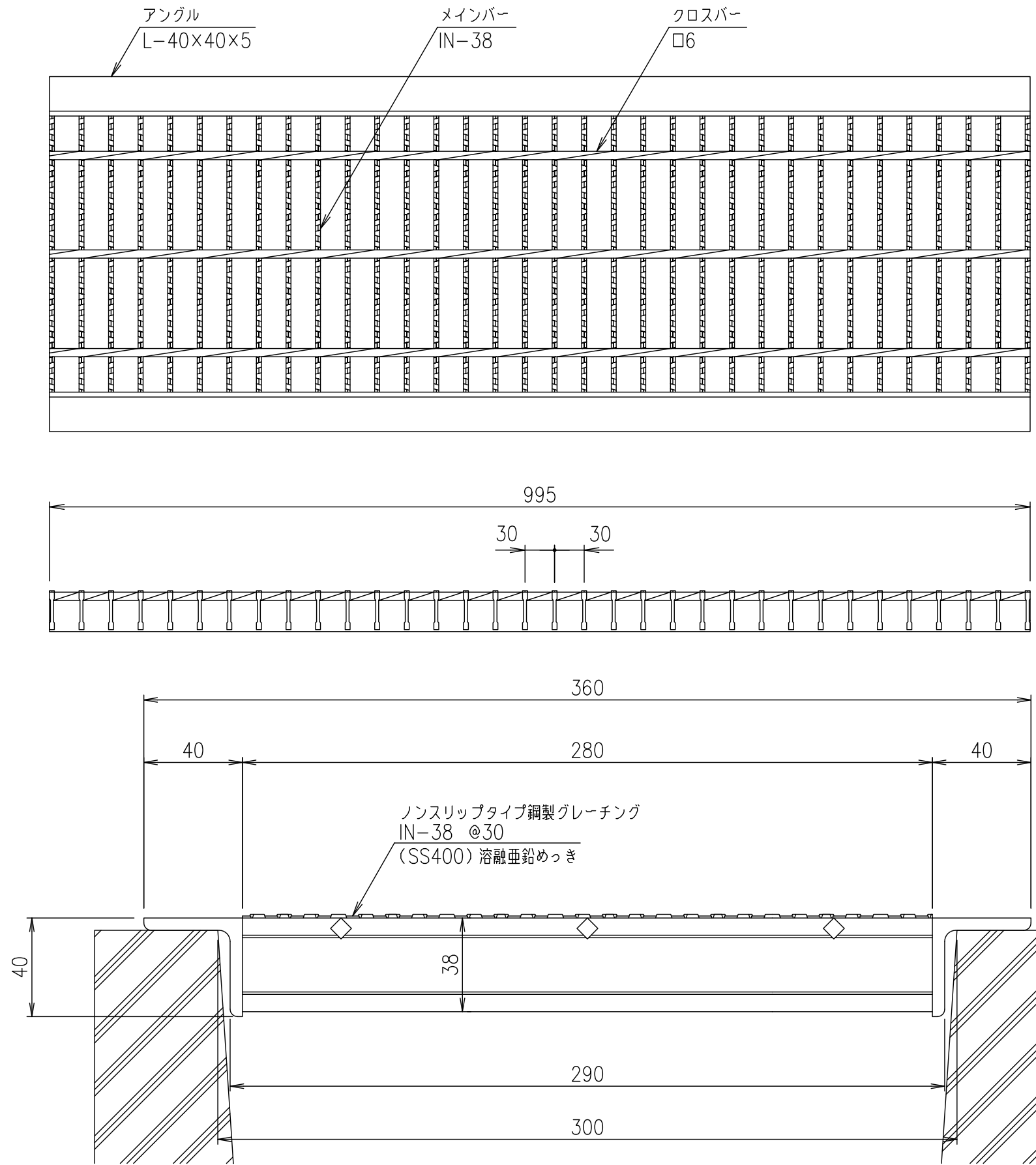
断面詳細図 S=1/2
