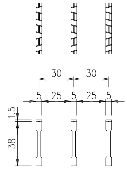
メインバー詳細図 S=1/2
