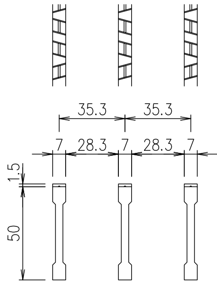
メインバー詳細図 S=1/2
