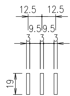
メインバー詳細図 S=1/2
