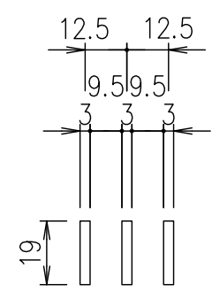
メインバー詳細図 S=1/2
