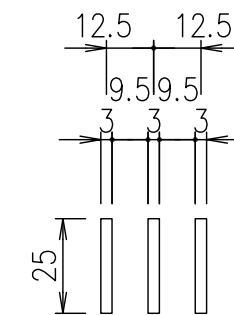
メインバー詳細図 S=1/2
