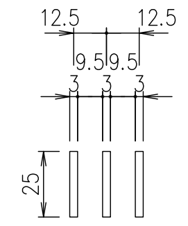
メインバー詳細図 S=1/2
