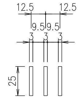
メインバー詳細図 S=1/2
