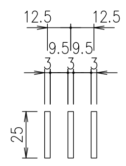
メインバー詳細図 S=1/2
