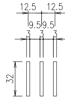
メンバー詳細図 S=1/2
