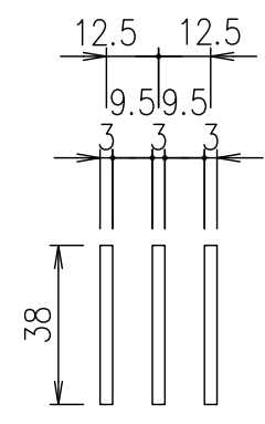
メインバー詳細図 S=1/2
