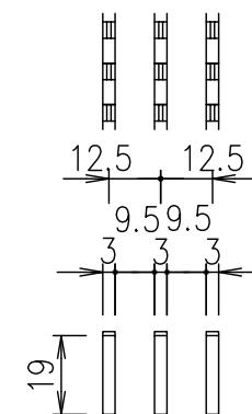
メインバー詳細図 S=1/2
