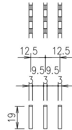
メインバー詳細図 S=1/2
