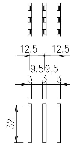
メインバー詳細図 S=1/2
