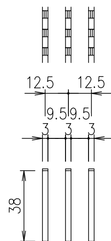
メインバー詳細図 S=1/2
