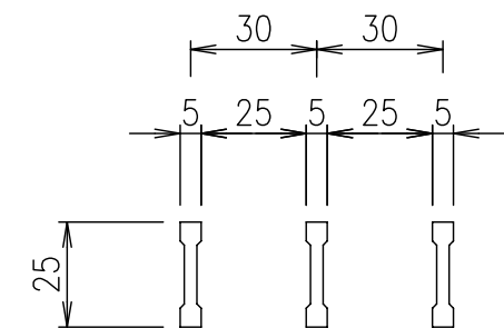
メインバー詳細図 S=1/2
