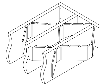
スベリ止め詳細図
