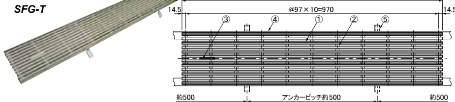
SFG-TF (補強タイプ)
