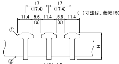
●メインバー詳細図
