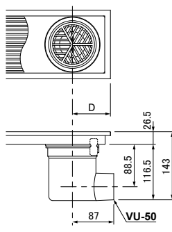
非防水横引き
