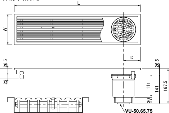
非防水縦引き
