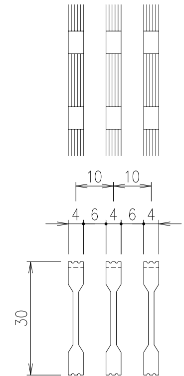
メンバーピッチ詳細図 S=1/1
