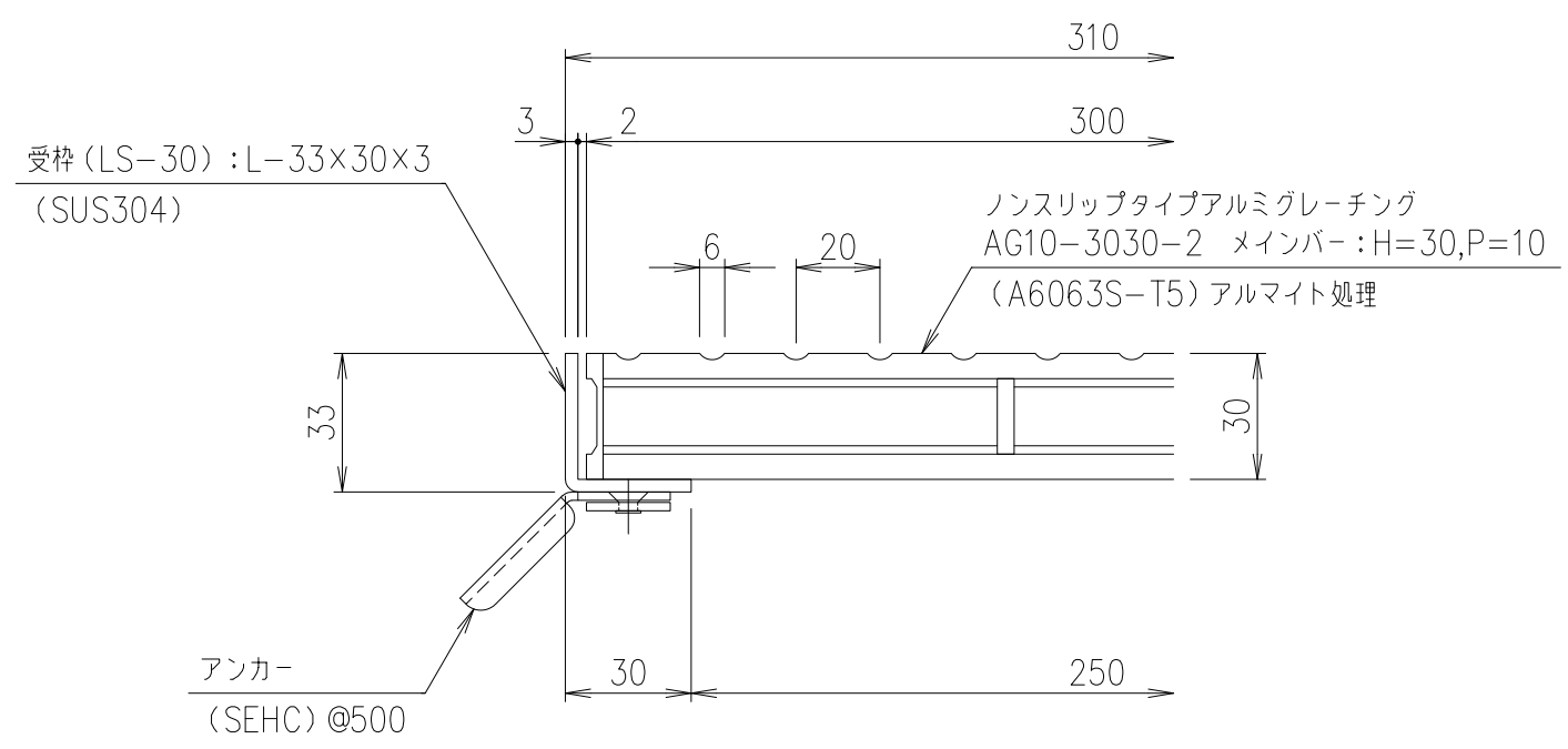
受枠 断面詳細図 S=1/2
