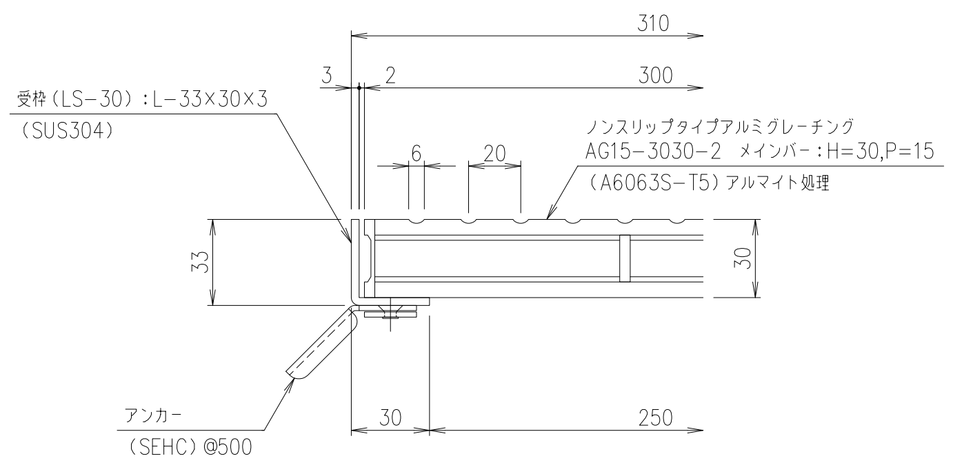
受棒 断面詳細図 S=1/2
